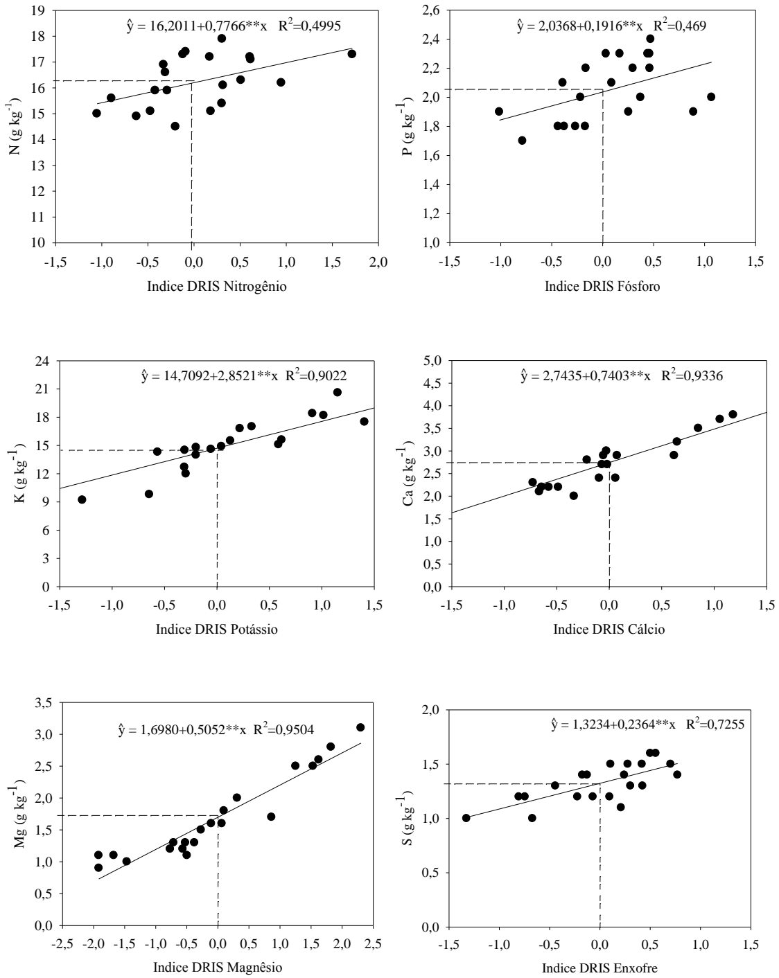
Figura 7. Relação entre os teores de macronutrientes na população de referência dos talhões de cana-soca de primeiro ano e seus respectivos índices DRIS (I DRIS), gerados com a norma 1.
