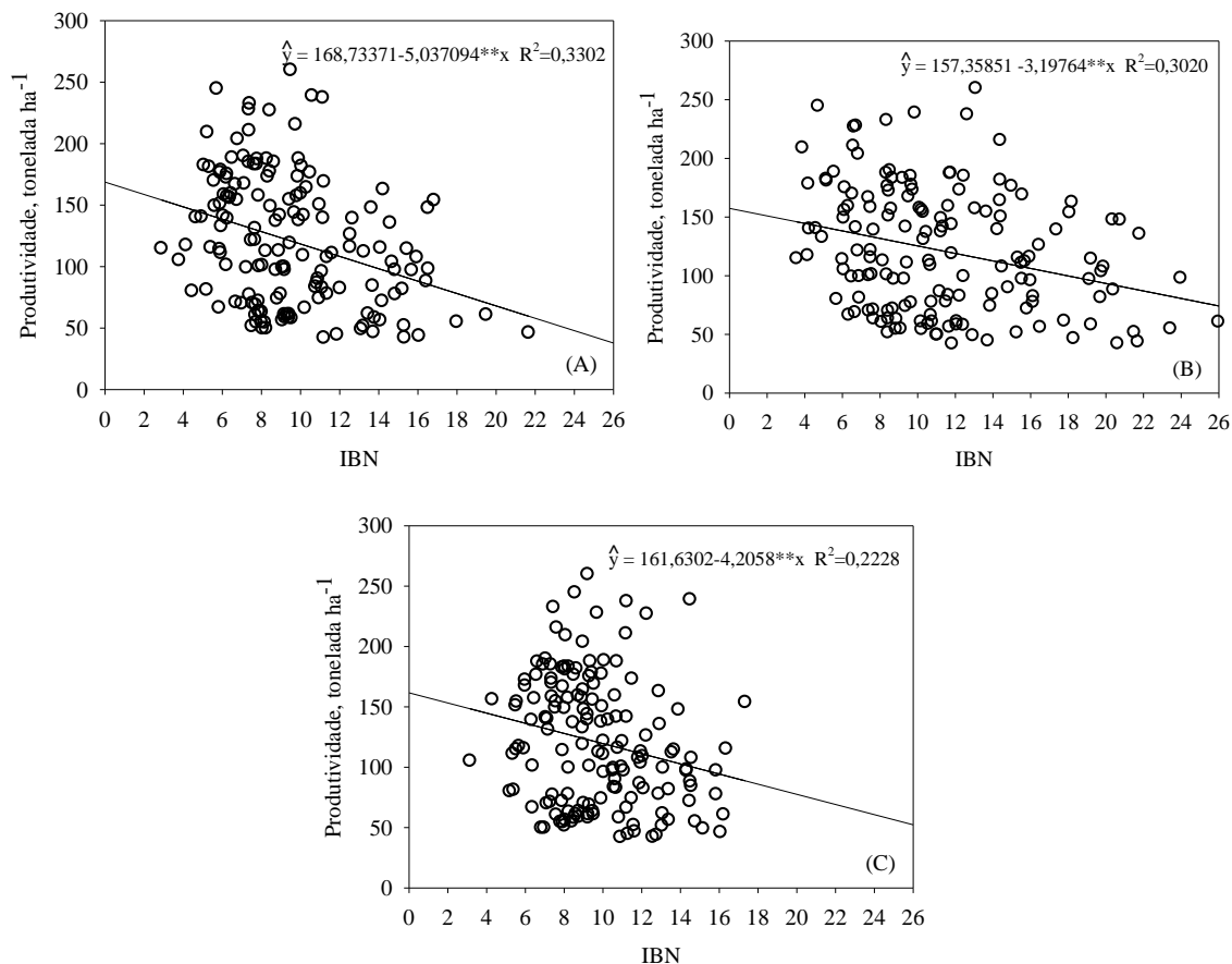
Figura 6. Relação entre índice de balanço nutricional e produtividade do banco de dados da cana-soca primeiro e segundo ano, por meio da utilização de 3 normas DRIS; (A) normas geradas com a cana-soca primeiro ano, (B) normas geradas com a cana-soca segundo ano, (C) normas geradas com a combinação da cana-soca primeiro e segundo ano.
